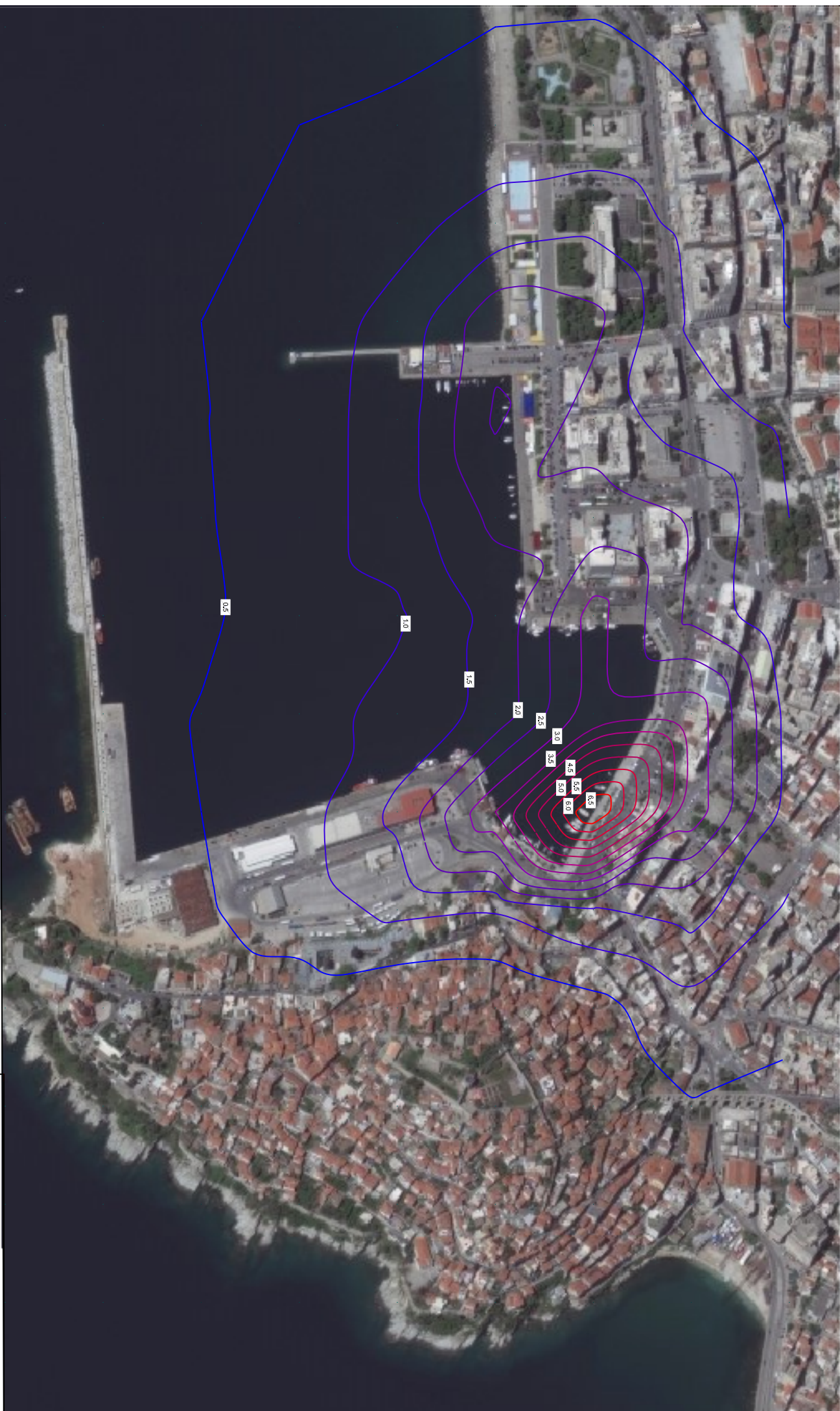
ΣΧΕΔΙΟ 5Α-1: ΕΚΤΙΜΩΜΕΝΗ ΣΥΓΚΕΝΤΡΩΣΗ CO2 (ppm) ΥΠΟΤΙΤΑΜΕΝΗ ΚΑΤΑΣΤΑΣΗ ΚΑΙΜ/ΚΑΛ: 1:30,000 ΣΦΡΑΓΙΔΑ - ΥΠΟΓΡΑΦΗ
